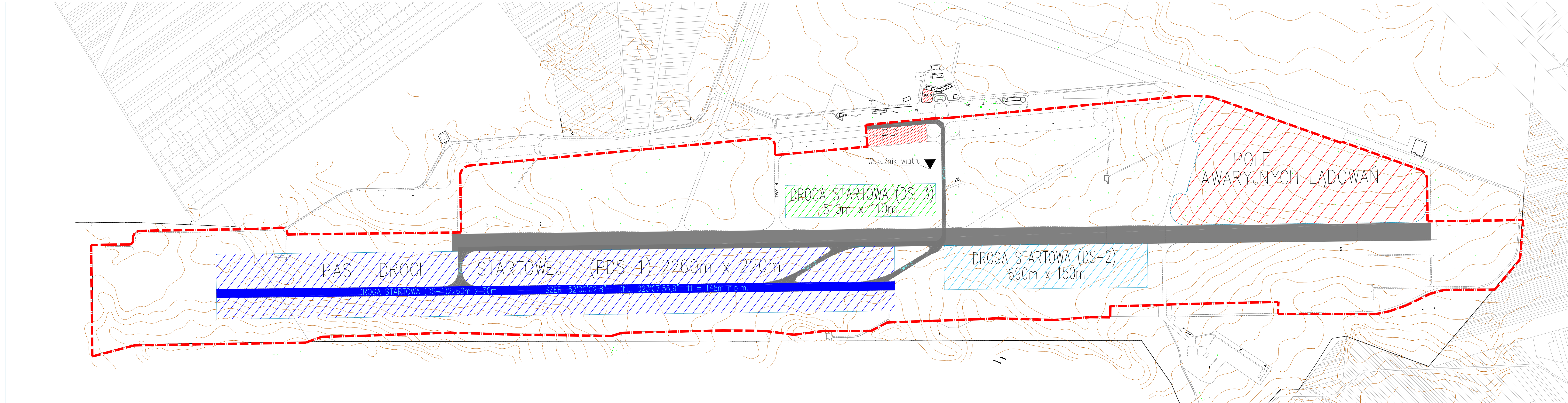
PLAN LĄDOWISKA BIAŁA PODLASKA skala 1:5000
